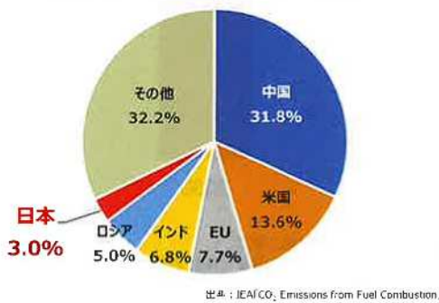
「世界のエネルギー起源CO 2 排出割合（2021年）」
