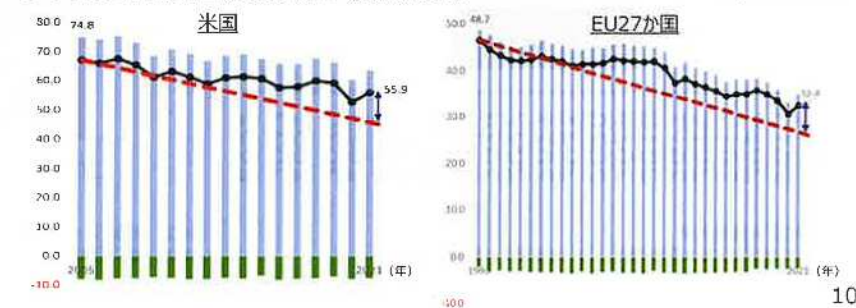
「参考：米国・EUの温室効果ガス排出・吸収量の推移」
